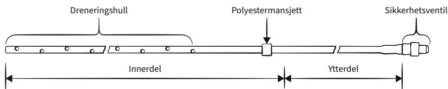
Figur: Skematisk fremstilling av et drainova® kateter
